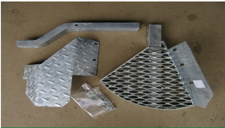
Lieferumfang: Tritthalter, Auftritt, Schutzblech, Auspuffschelle, Schraubensatz
